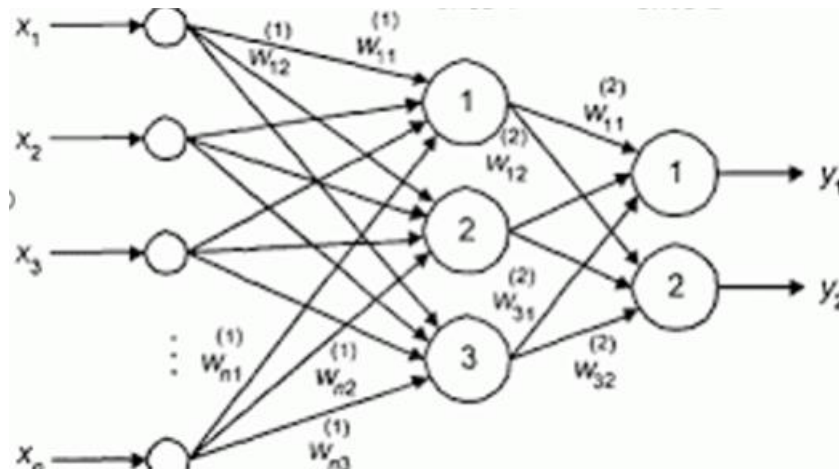
Рис. 2. Перцептрон
