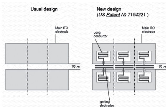
Рис.2. Дизайн прозорих електродів (до и після використання ТРІВЗ
